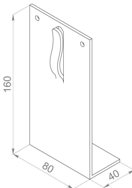
Консоль несущая 160
