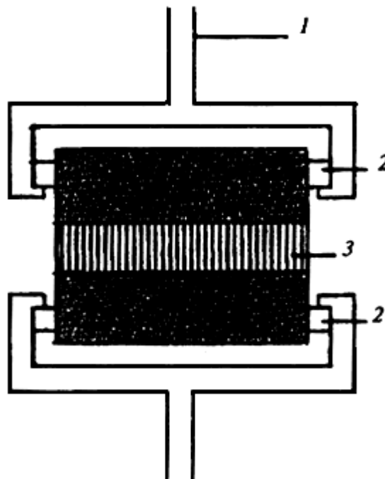
1 - хомут; 2 - опора; 3 - образец
